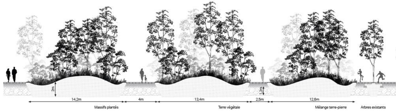
COUPE LONGITUDINALE
