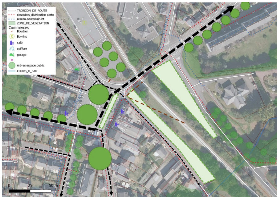
Schéma de principe du réaménagement de la place E. Herbert à Fougères (source : Cerema Ouest)
